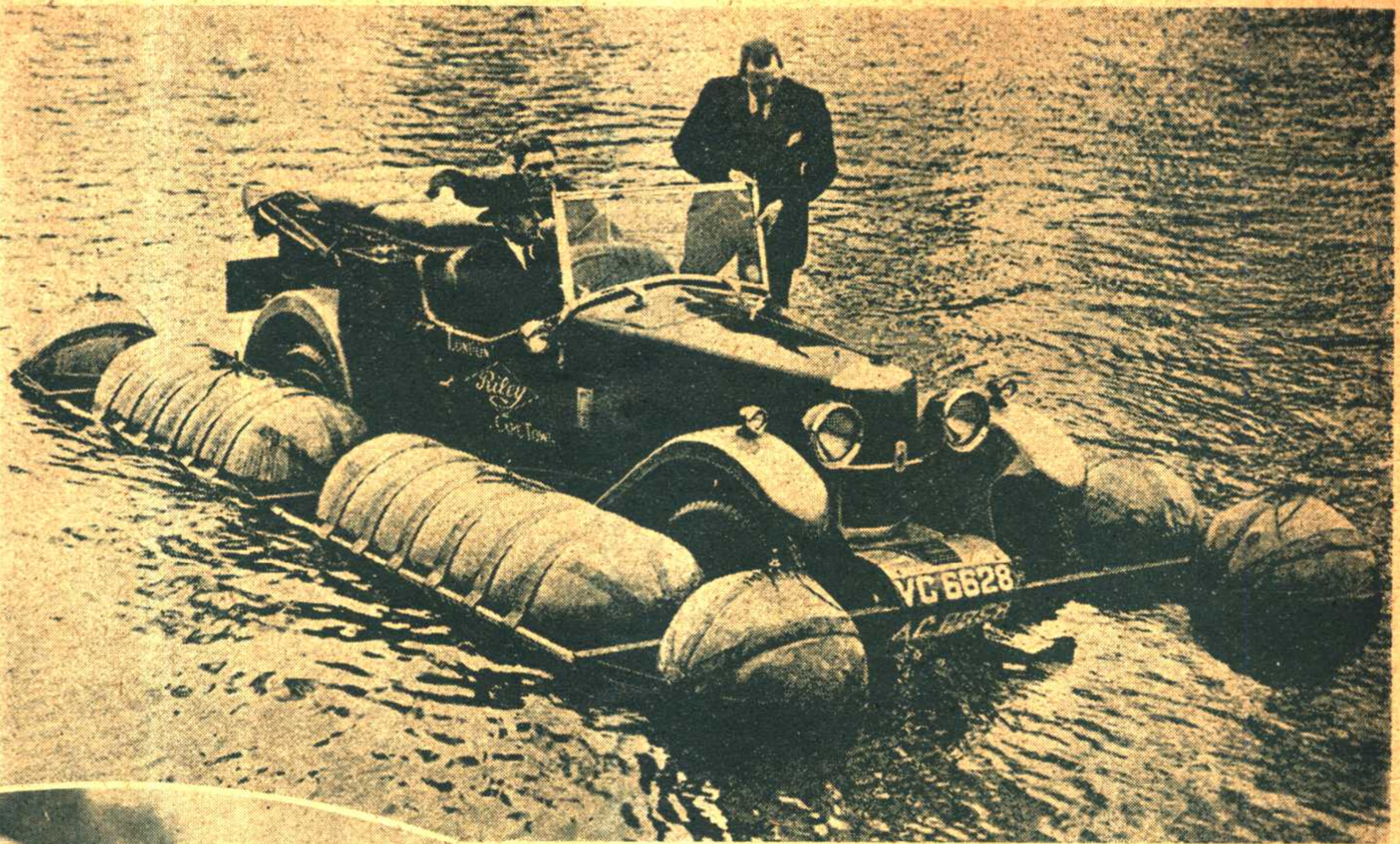
(上) 水陸兩用汽車 圖為萊里一 三·九馬力之汽車，車輪比較普通者較 大，周圍附以浮囊，後方有鋼鐵所製之 推行機，在水上亦可以隨意進行。
