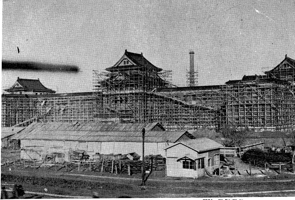
工程を急ぐ關東軍司令部應舎 設計 軍經理部 施工 大林組
