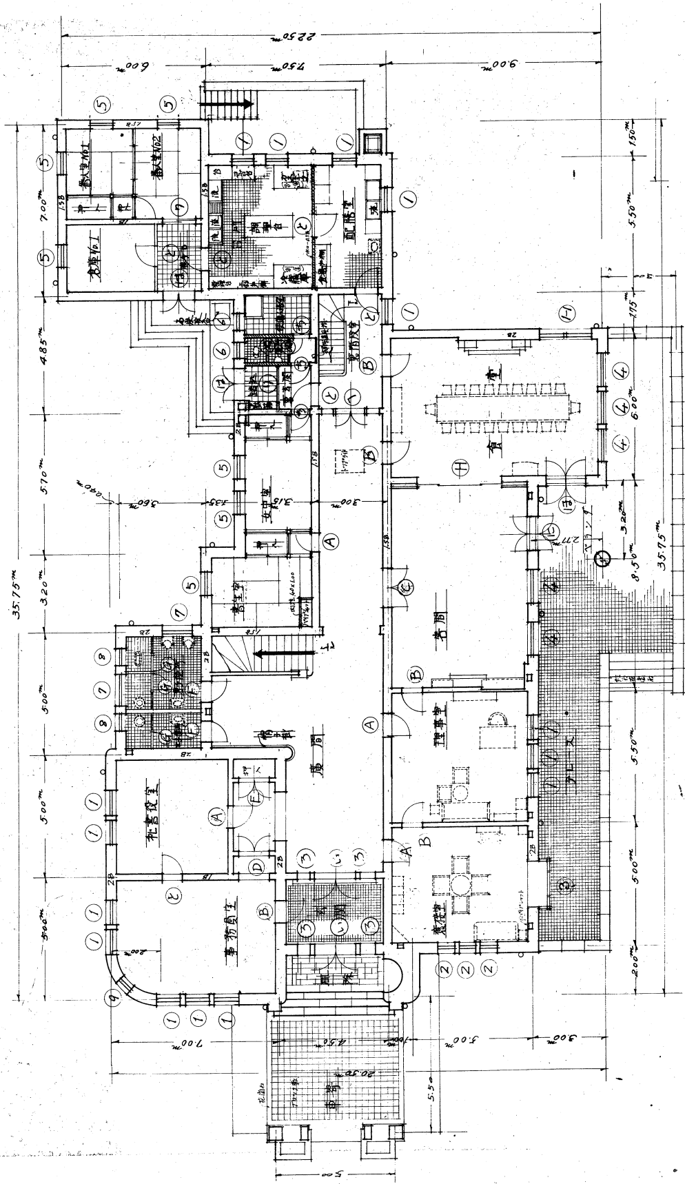
滿鐵新京理事公館 = 1 階平面
