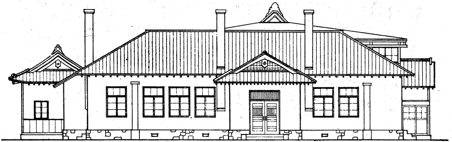
正面圖
