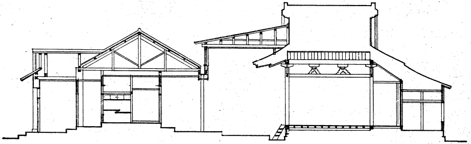
縱斷面圖
