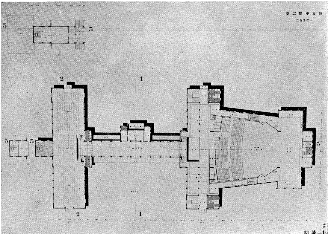
壹等 (E) 1階 (下) 2階平面圖
