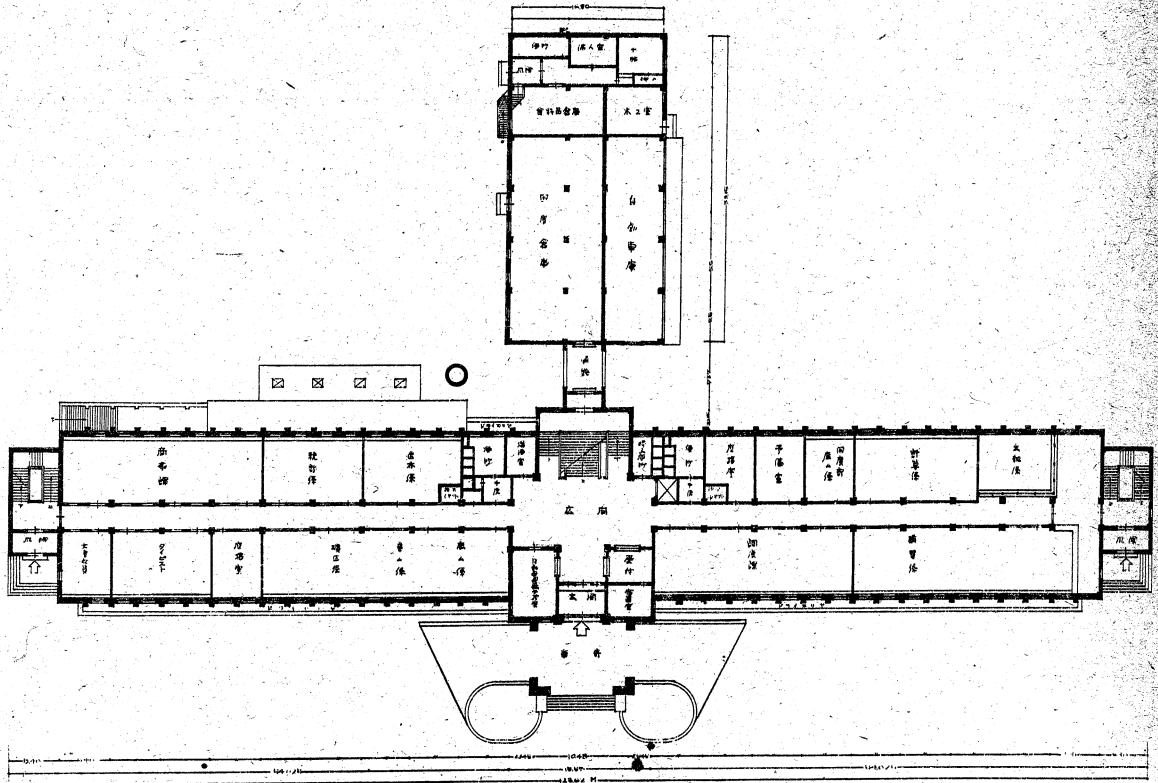
滿洲炭礦株式會社本社平面圖
