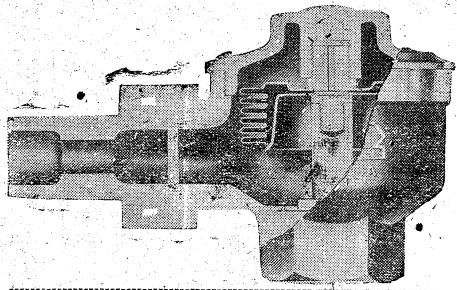
BN 914-A型 スチーム トラップ
