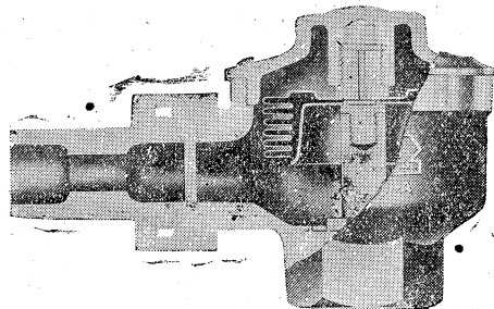
BN 914-A型 スチーム トラップ
